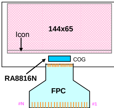
Figure A-1 : COG Module
